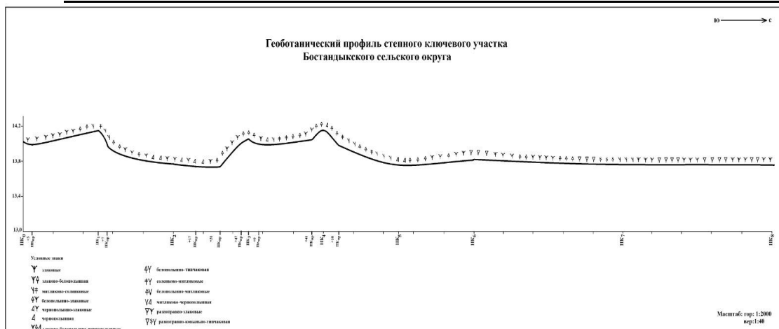
Рисунок - 2 - Геоботанический профиль, Бостандыкского ключевого участка.
