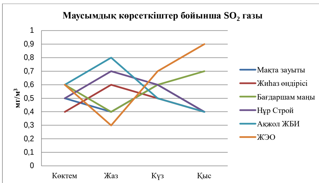
2-сурет- Маусымдық көрсеткіштер бойынша \text{SO}_2 газы
