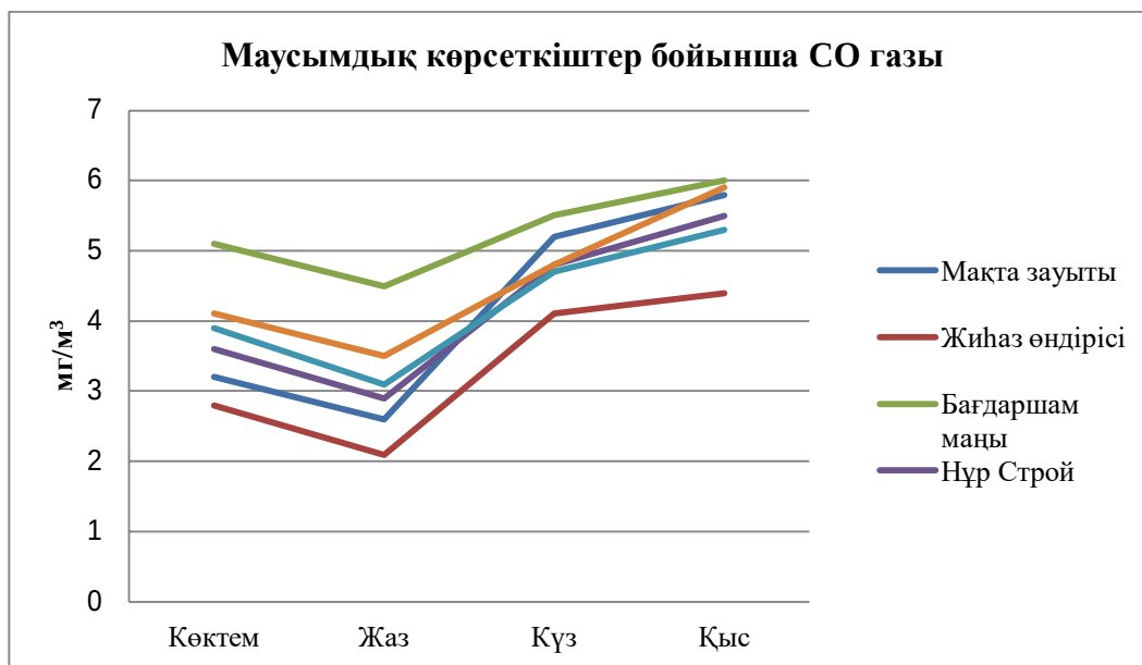
1- сурет- Маусымдық көрсеткіштер бойынша \text{CO} газы
